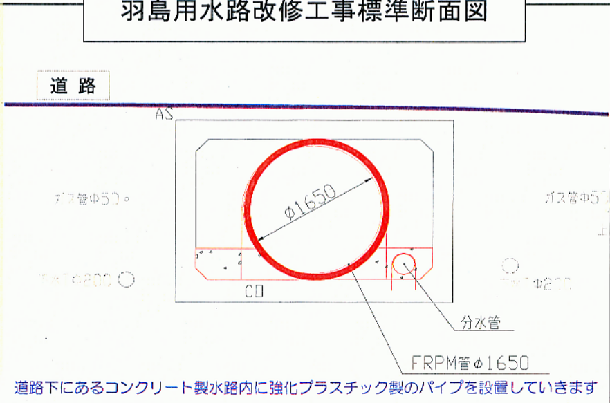
羽島用水路改修工事標準断面図
